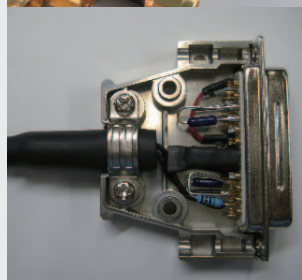
ハーネス加工例
